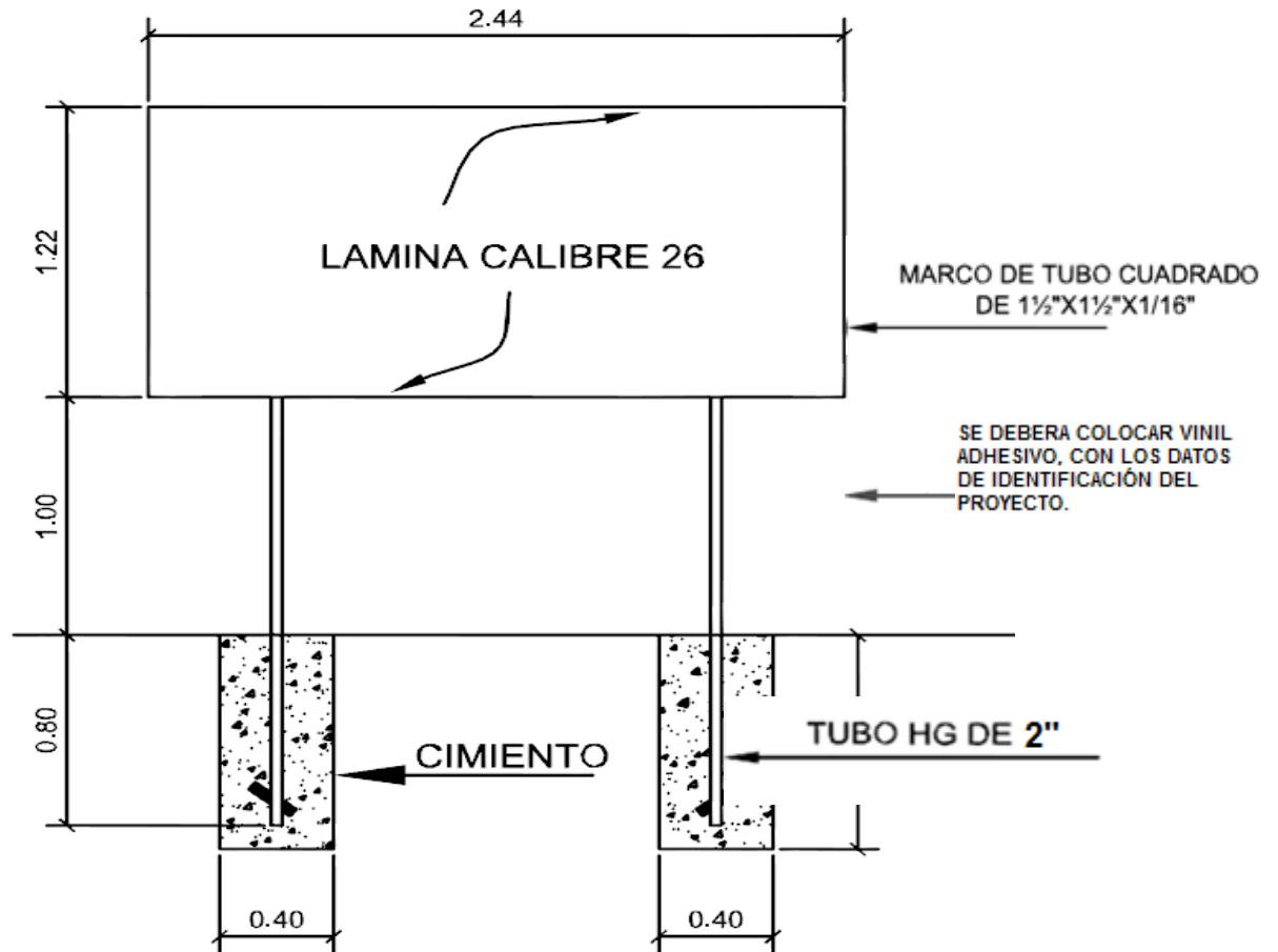
ELEVACIÓN FRONTAL
